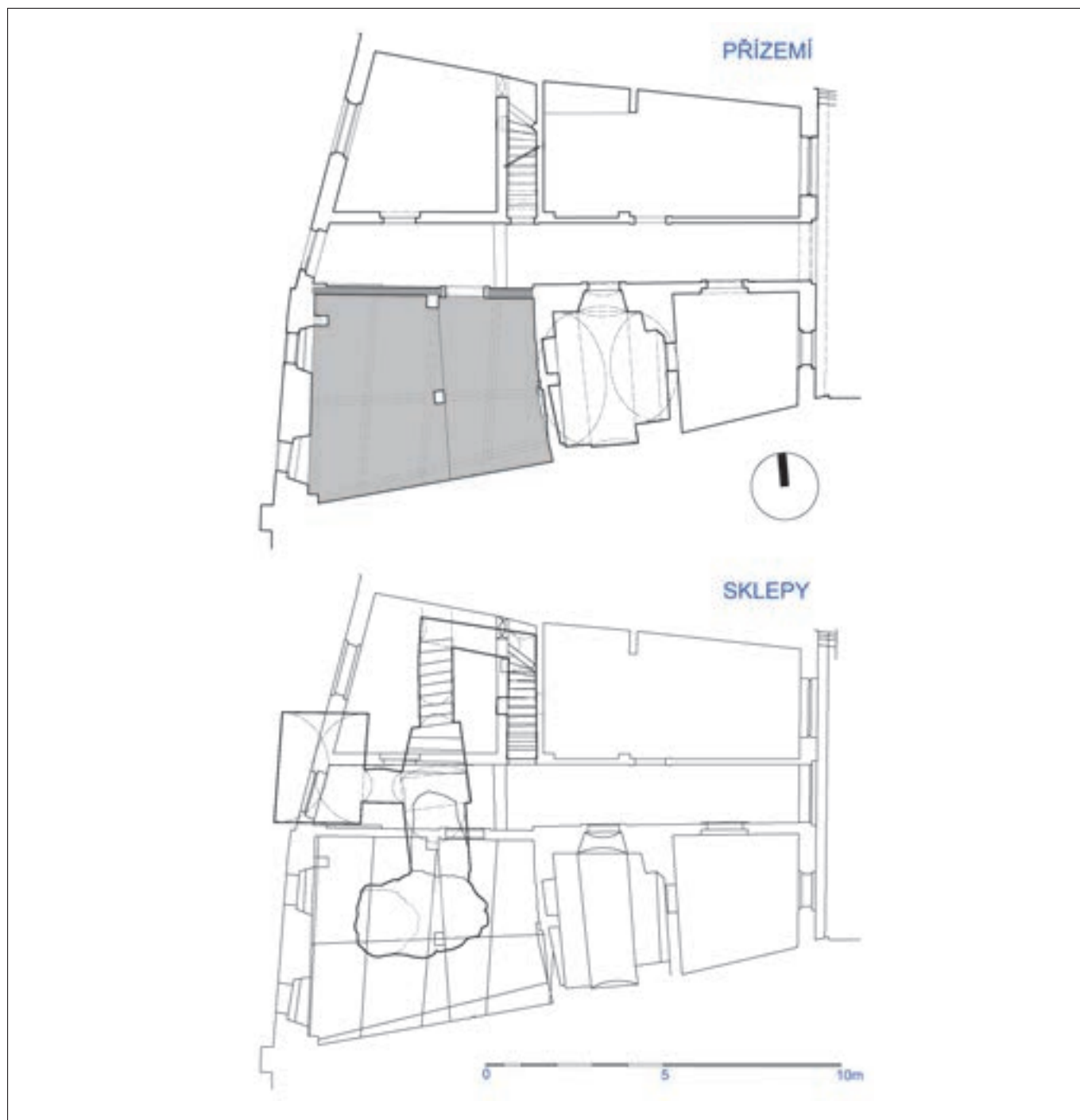
Kouřim (okres Kolín) – Dubová ulice, dům čp. 63. Půdorysné plány zaměření současného stavu. Šedě jsou vyznačeny dochované dřevěné konstrukce roubené stěny a záklopového stropu, datované dendrochronologicky do roku 1693 (zaměření a kresba J. Veselý).
