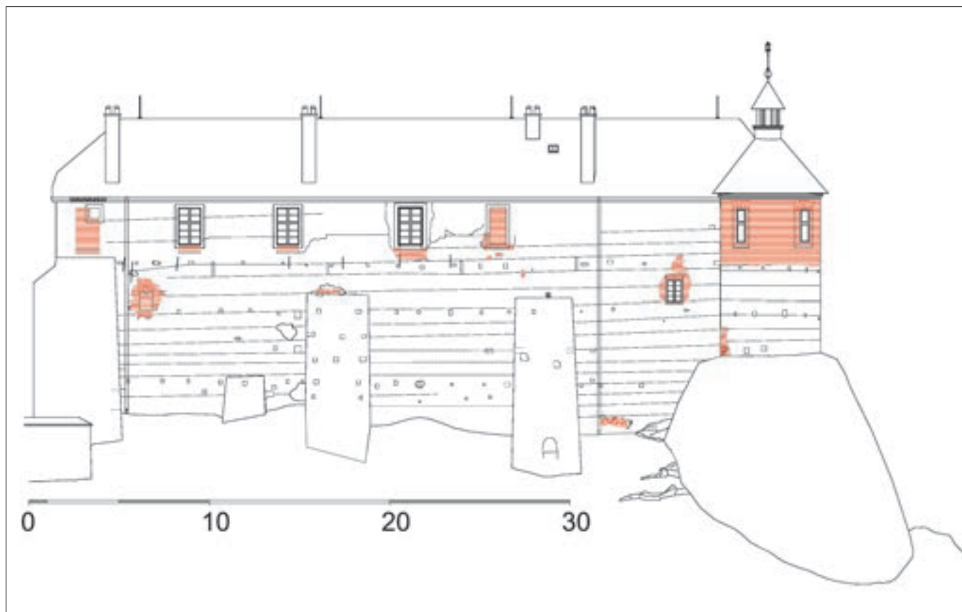
Český Šternberk (okres Benešov) – brad čp. 1. Zaměření severozápadní fasády dolního bradu, zachycující všechny podstatné nálezo- vé situace odbalené po celoplošném sejmutí poškozených omítek. Průzkum umožnil určit rozsah středověkého zdiva, identifikovat čtveřici zaslepených střel a řadu dalších podrobností. Plošné odstranění starších omítek na památkových objektech je vnímáno jako nežádoucí. Přesto se mu občas nelze vyhnout. Je pak namístě maximálně využít příležitosti k poznání a podrobné dokumentaci všech stop historického i konstrukčního vývoje stavby (zaměření J. Veselý a J. Kypťá; kresba J. Veselý, 2014 a 2015).
