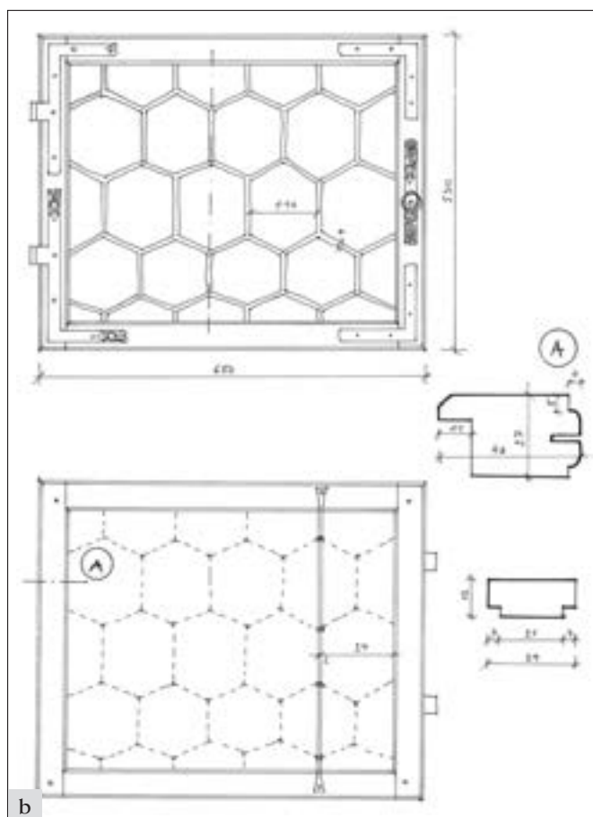
Březnice (okres Příbram), areál panského pivovaru čp. 30 a 31: a – barokní okno (patrně z doby výstavby pivovaru ve 20. letech 18. století) zachované ve východní fasádě blavního křídla v 1. patře sladovny za hvozdem. Pobléd na okenní výplň z interiéru; b – výkres poblédu na barokní okenní rám a okenní horní levé křídlo v měřítku 1 : 10; c – detail profilace rámu okna i křídla; d – poutce, obrtlíku, vnějšího závěsu a středového štítiku s kroužkem v měřítku 1 : 1 (foto a kresba D. Havlíková).
