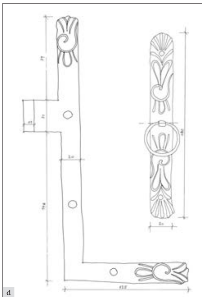
Březnice (okres Příbram), areál panského pivovaru čp. 30 a 31: a – barokní okno (patrně z doby výstavby pivovaru ve 20. letech 18. století) zachované ve východní fasádě blavního křídla v 1. patře sladovny za hvozdem. Pobléd na okenní výplň z interiéru; b – výkres poblédu na barokní okenní rám a okenní horní levé křídlo v měřítku 1 : 10; c – detail profilace rámu okna i křídla; d – poutce, obrtlíku, vnějšího závěsu a středového štítiku s kroužkem v měřítku 1 : 1 (foto a kresba D. Havlíková).
